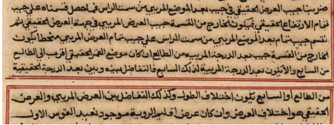
Figure 3. Zīj-i Sultānī text: calculation of the latitude and longitude parallax of the Moon
